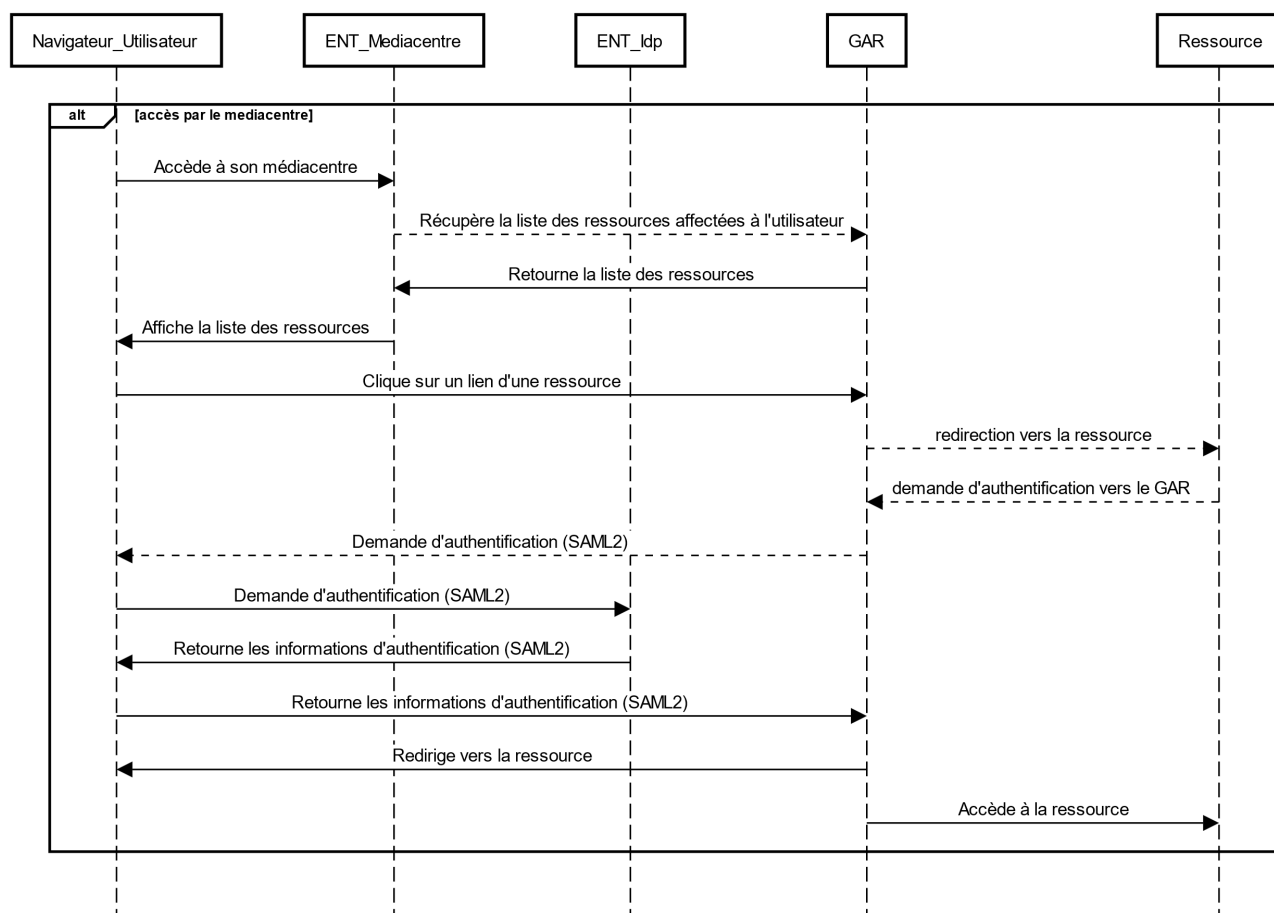
Figure 9 - Médiacentre dans le processus d'accès aux ressources (exemple en SAML)
