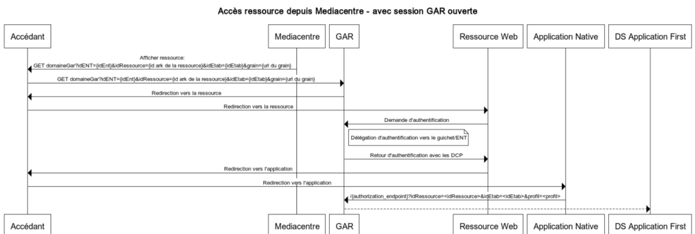
Figure 7 - Accès depuis le médiacentre avec une session GAR ouverte
