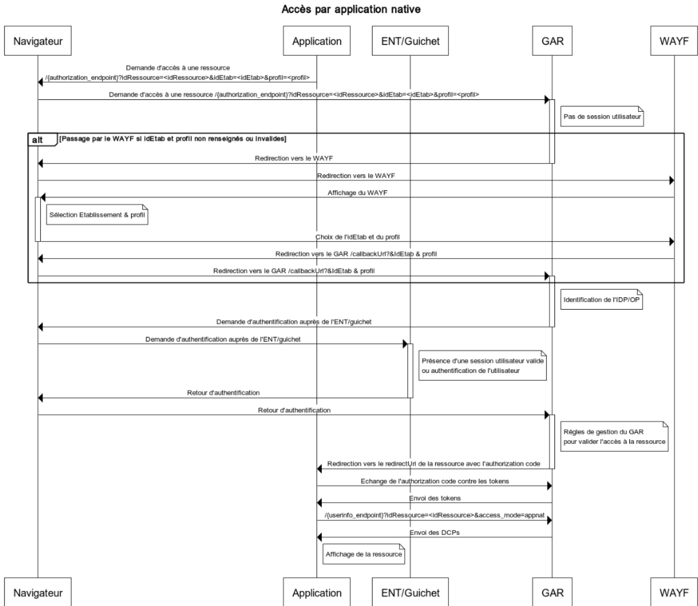
Figure 5 - Diagramme de séquence - Accès par application native
